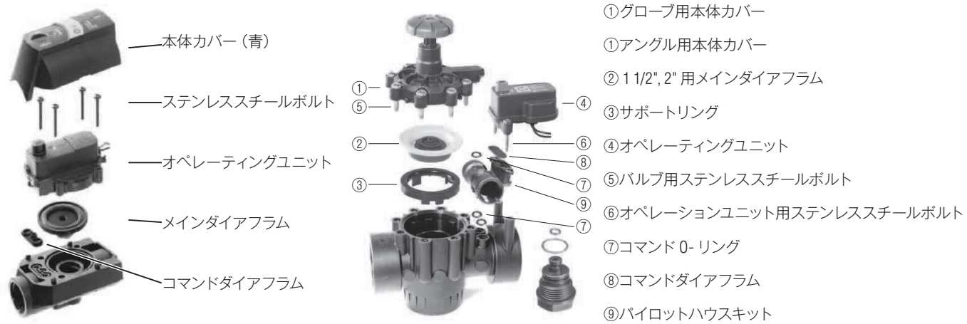
分解図
